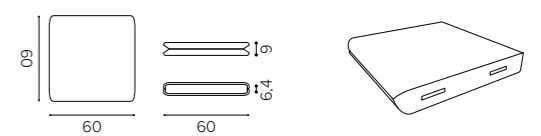
MP TRE2 double central table with power supply tavolino centrale doppio con elettrificazione
