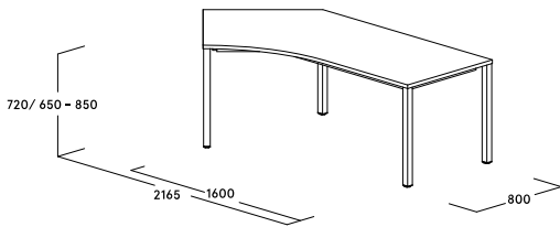
Freiformtisch links oder rechts
