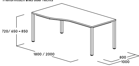
Freiformtisch links oder rechts
