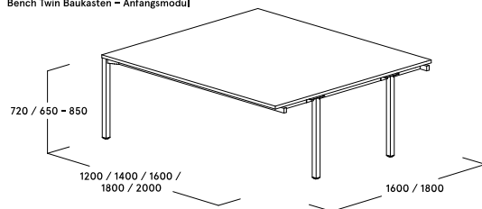
Bench Twin Baukasten – Mittelmodul
