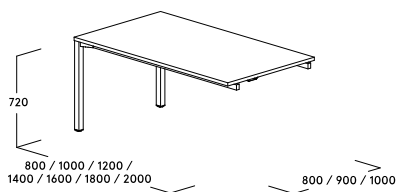
Anbautisch für Konferenztisch
